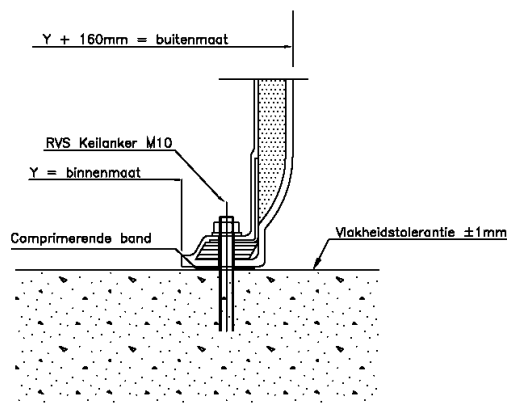
Detail: Funderingaansluiting
