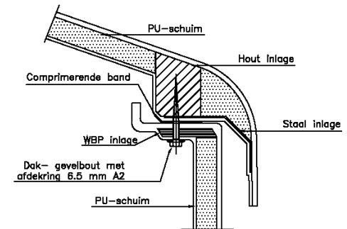
Detail: Dakaansluiting
