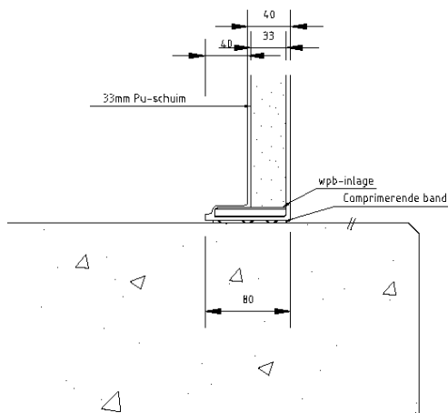
Detail: Funderingaansluiting
